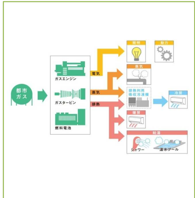
コージェネレーションシステム概略図
